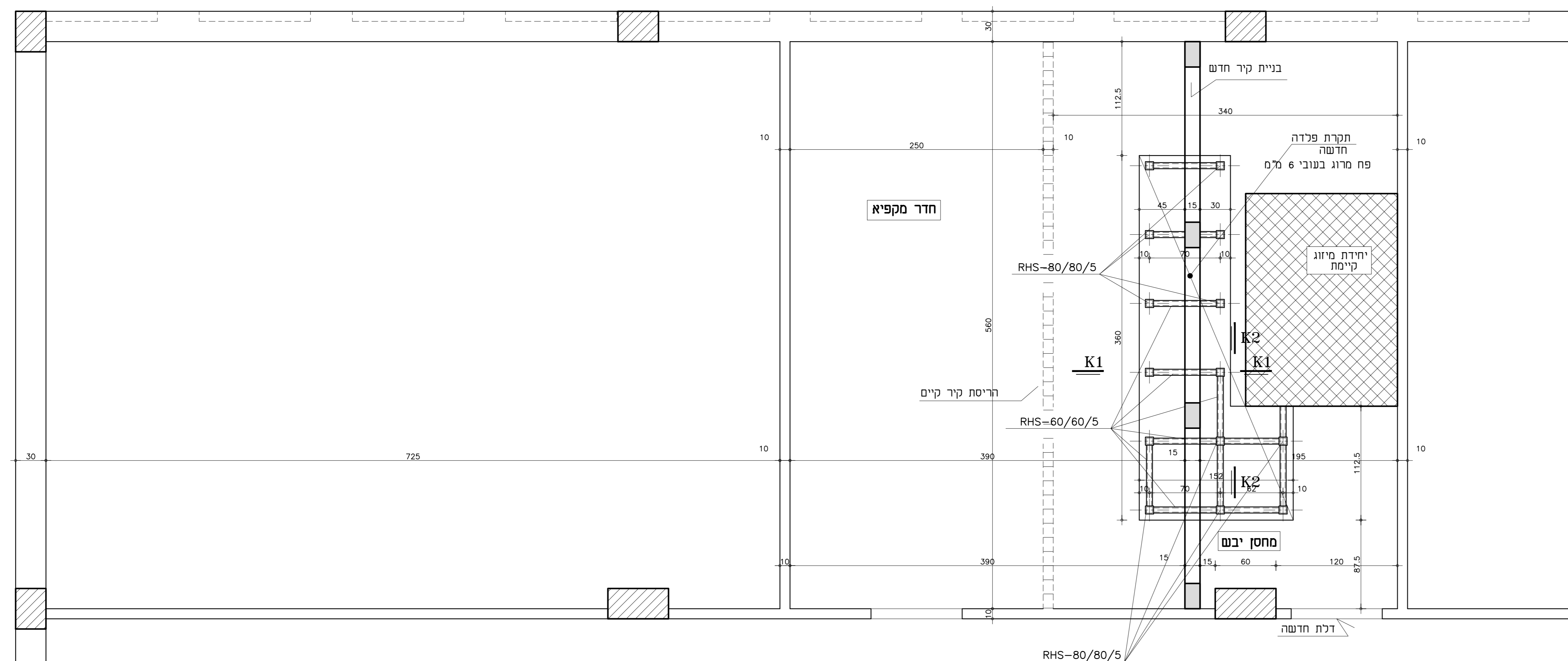
תוכנית משטח פלדה
